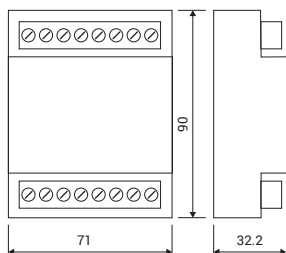
DALI-4CV (L406MA0GT4A03) DALI-4CC (L405MA0GC4A03)
